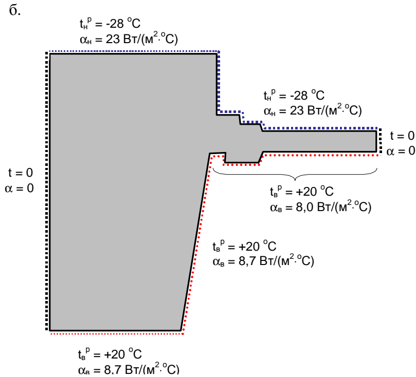
Рис.Г2. Расчетная схема (а) и схема задания граничных условий (б) узла примыкания оконного блока к оконному проему: 1 – кирпичная кладка - \lambda_{\text{Б}} = 0,8 \text{ Вт}/(\text{м} \cdot ^{\circ}\text{C}) ; 2 – цементно-песчаный раствор - \lambda_{\text{Б}} = 0,93 \text{ Вт}/(\text{м} \cdot ^{\circ}\text{C}) ; 3 – древесина поперек волокон - \lambda_{\text{Б}} = 0,22 \text{ Вт}/(\text{м} \cdot ^{\circ}\text{C}) ; 4 – монтажная пена - \lambda_{\text{Б}} = 0,05 \text{ Вт}/(\text{м} \cdot ^{\circ}\text{C}) ; 6 –экструдированный пенополистирол - \lambda_{\text{Б}} = 0,05 \text{ Вт}/(\text{м} \cdot ^{\circ}\text{C}) ; 7- стекло - \lambda_{\text{Б}} = 0,76 \text{ Вт}/(\text{м} \cdot ^{\circ}\text{C}) ; 8 – воздушная прослойка 12 мм - \lambda_{\text{эКВ}} = 0,08 \text{ Вт}/(\text{м} \cdot ^{\circ}\text{C}) ; 9 – алюминий - \lambda = 220 \text{ Вт}/(\text{м} \cdot ^{\circ}\text{C}) ; 10 – герметик - \lambda_{\text{Б}} = 0,34 \text{ Вт}/(\text{м} \cdot ^{\circ}\text{C}) ; 11 – пароизоляционная лента - \lambda_{\text{Б}} = 0,56 \text{ Вт}/(\text{м} \cdot ^{\circ}\text{C}) ;
